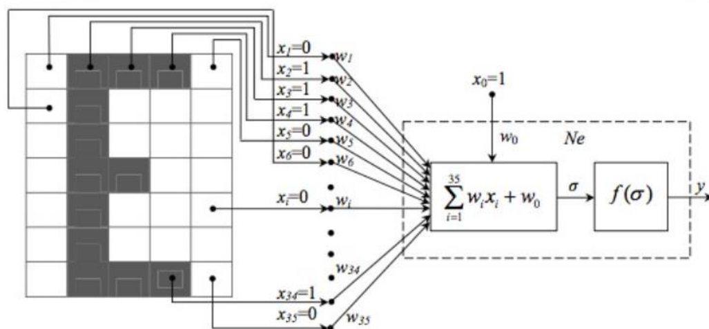
Расми 2. Одитарин шабакаи нейронӣ (персептрон) барои шинохти тасовир (ҳарф).
