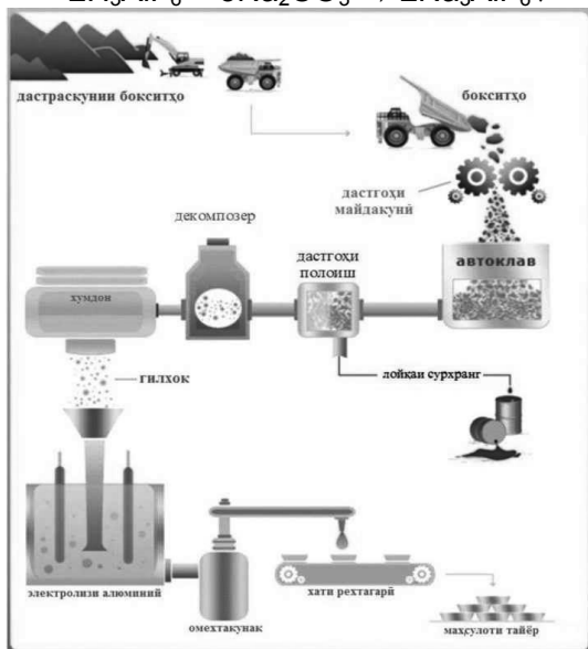
Нақшаи умумии истеҳсоли алюминий
