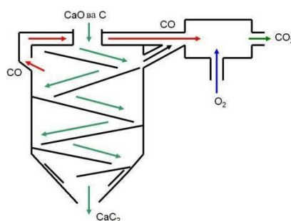
Хумдон барои истеҳсоли карбиди калсий
