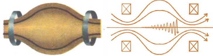
Расми 2. Нақша ва сохти зоҳирии доми магнитии кушод (Пробкатрон).
