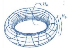
Расми 6. Тарҳи стелларатор (Тамоили плазма дар доми тороидалӣ)
