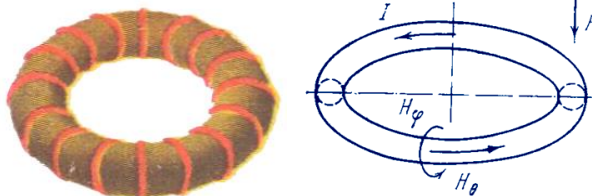
Расми 7. Нақшаи «Токомак»
