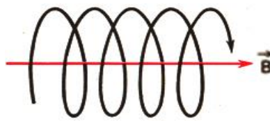
Расми 1. Масири ҳаракати зарраи заряднок дар майдони магнитӣ.
